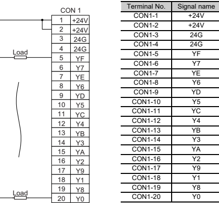
Câblage du connecteur pour sorties
