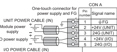
Câblage de connecteur pour alimentation et FG
