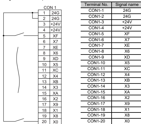
Câblage du connecteur pour entrée
